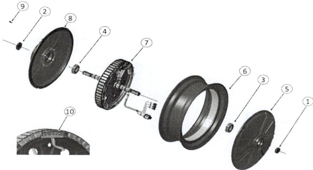
(Ảnh: Động cơ điện một chiều dùng cho xe mô tô điện, xe gắn máy điện, có vành sau DRT00007658)
